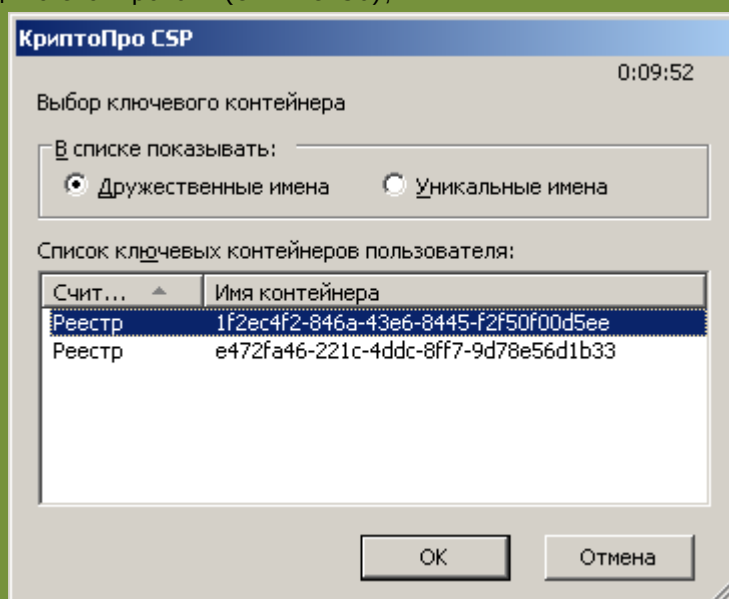
Рис. 205. Выбор ключевого контейнера
