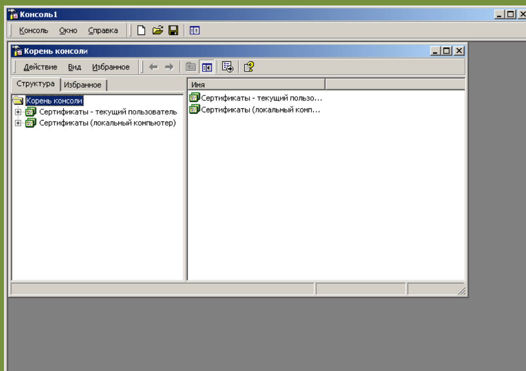
Рис. 54. Консоль MMC
