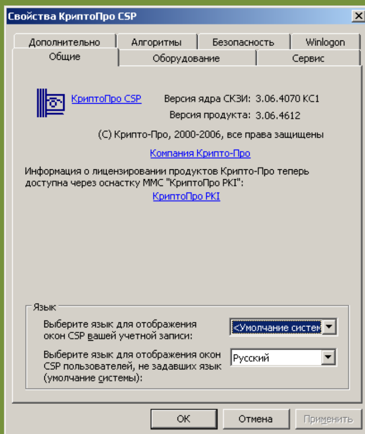
Рис. 5. Панель настройки
